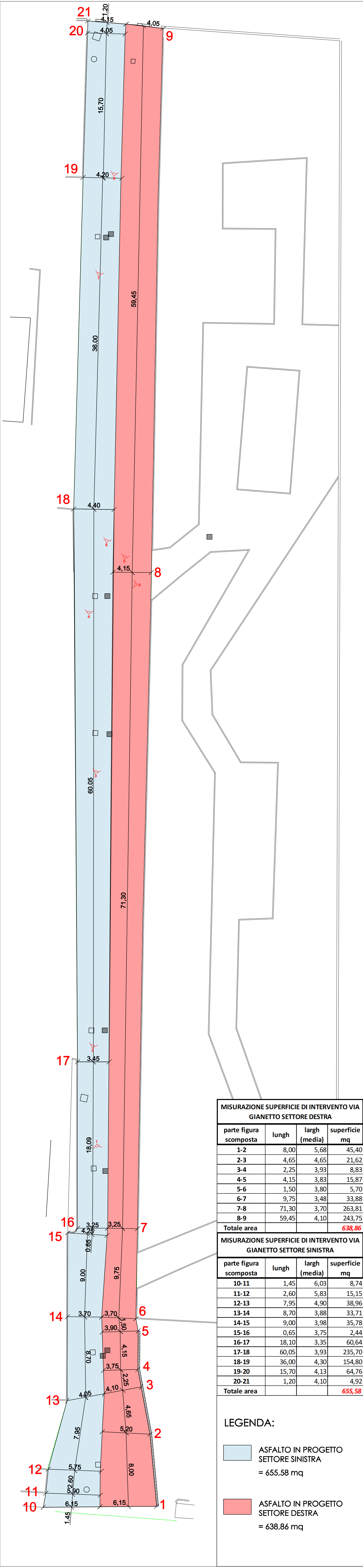
PLANIMETRIA SITUAZIONE IN PROGETTO
